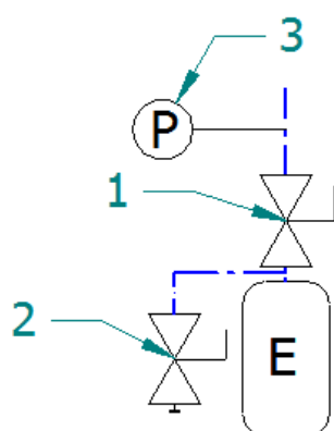
Obr 18: Zapojení expanzní nádoby
