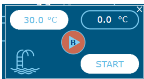
Obr 11: Okno bazénu
