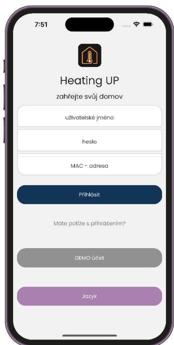
Obr 17: Přihlašovací stránka
