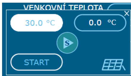
Obr 10: Okno soláru
