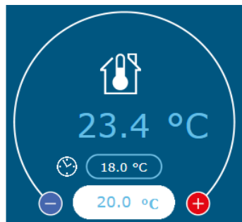
Obr 7: Nastavení teplot
