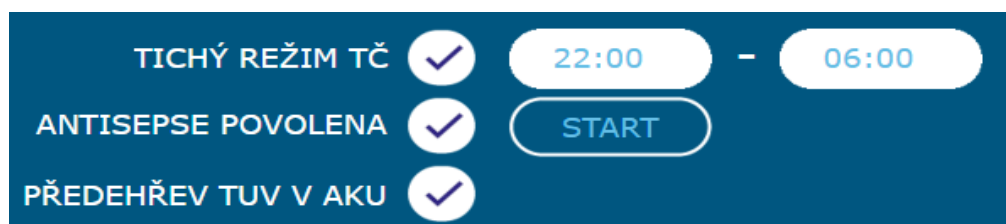
Obr 8: TUV – antiseptise
