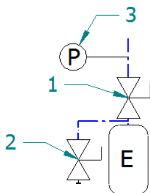
Obrázek 17: Zapojení expanzní nádoby
