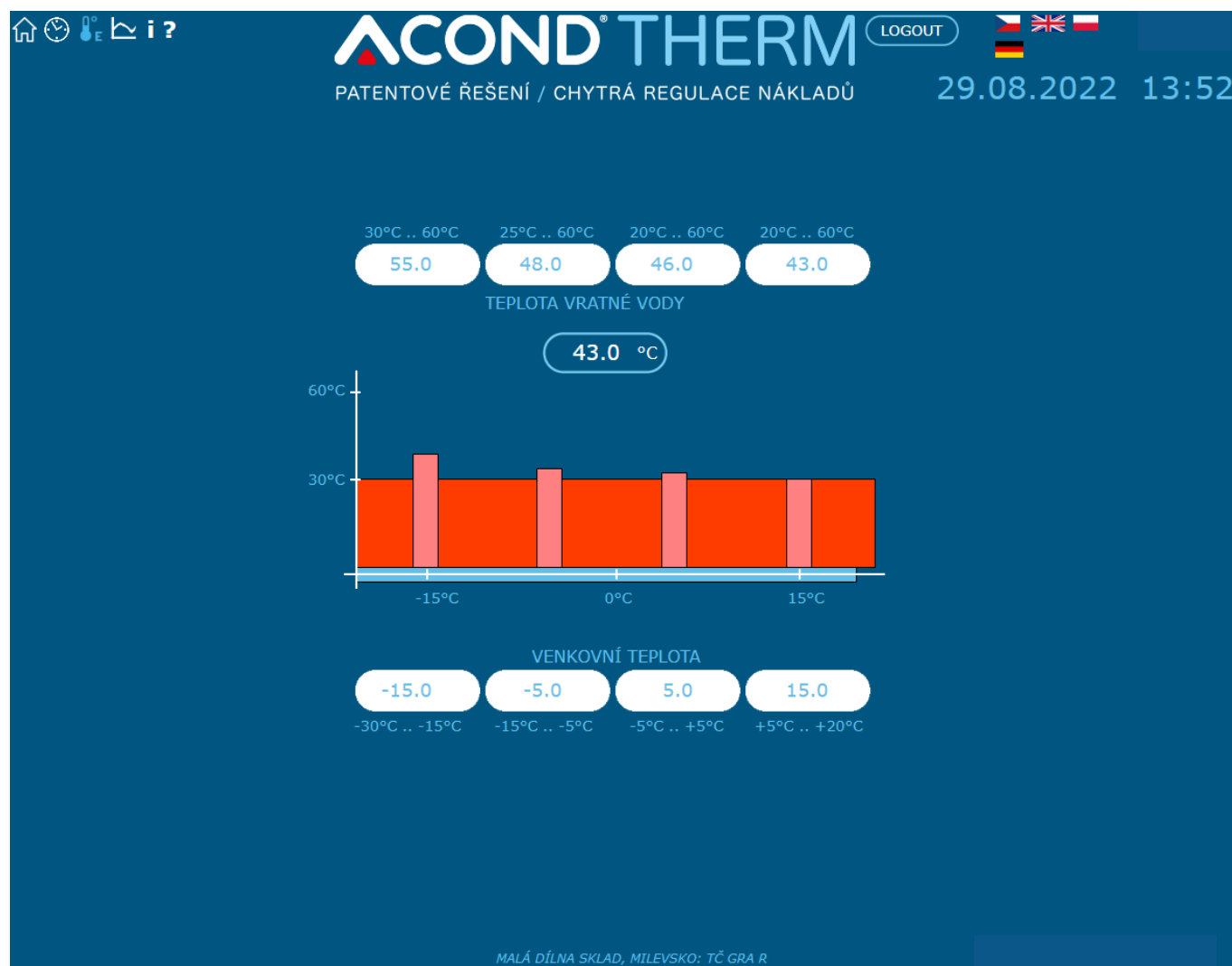
Obrázek 16: Nastavení ekvitermní regulace
